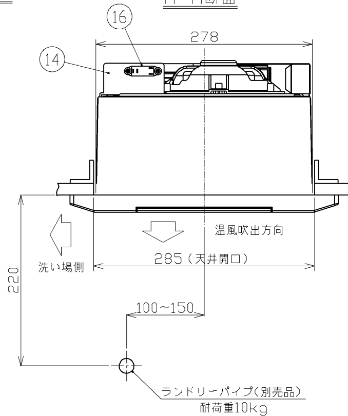
A-A断面
