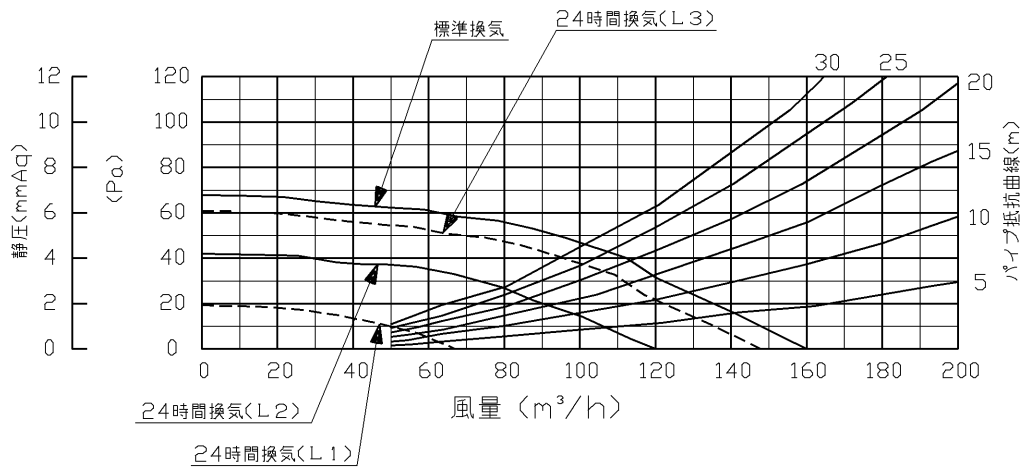
静圧風量特性曲線(換気運転時)
