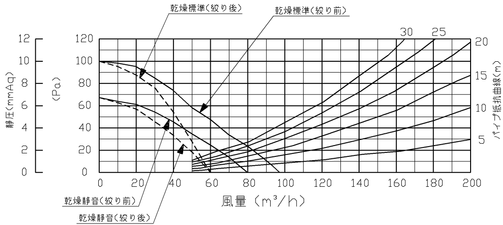
静圧風量特性曲線(乾燥運転時)
