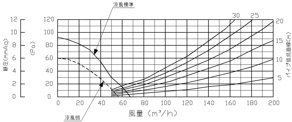
静圧風量特性曲線(涼風運転時)
