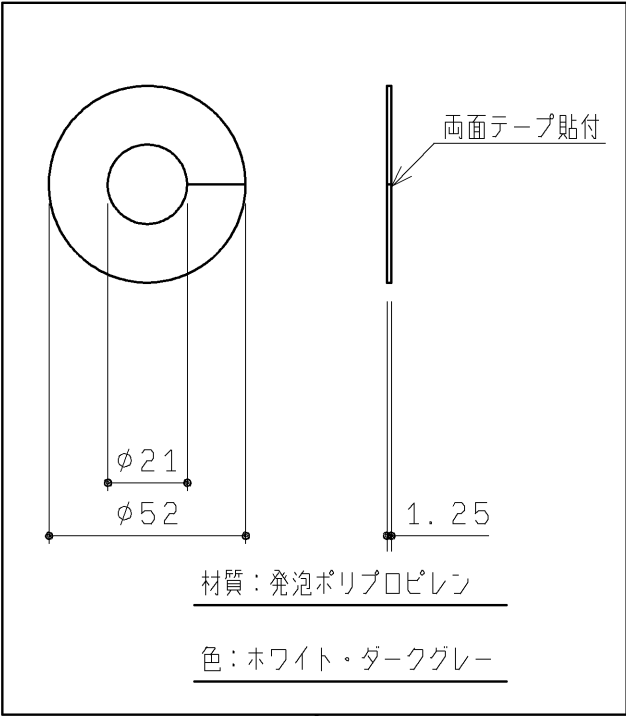
カバー（1ヶ）
