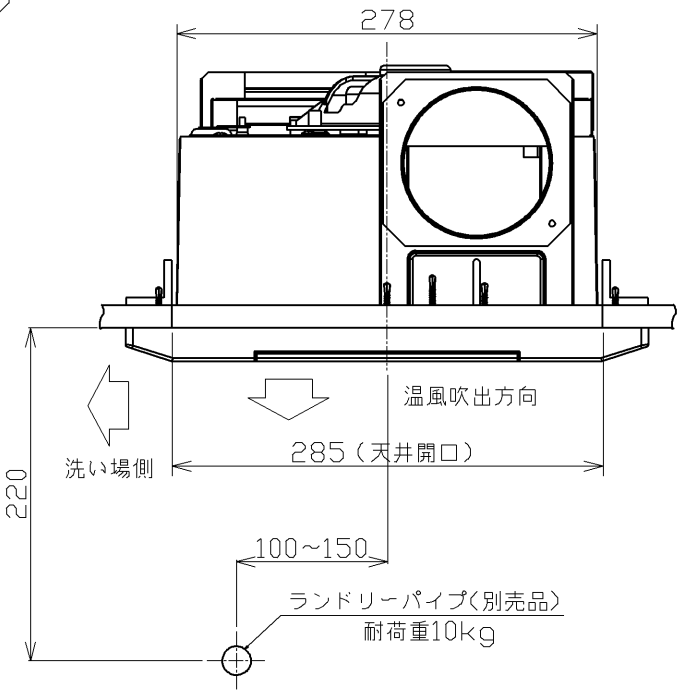
A-A断面
