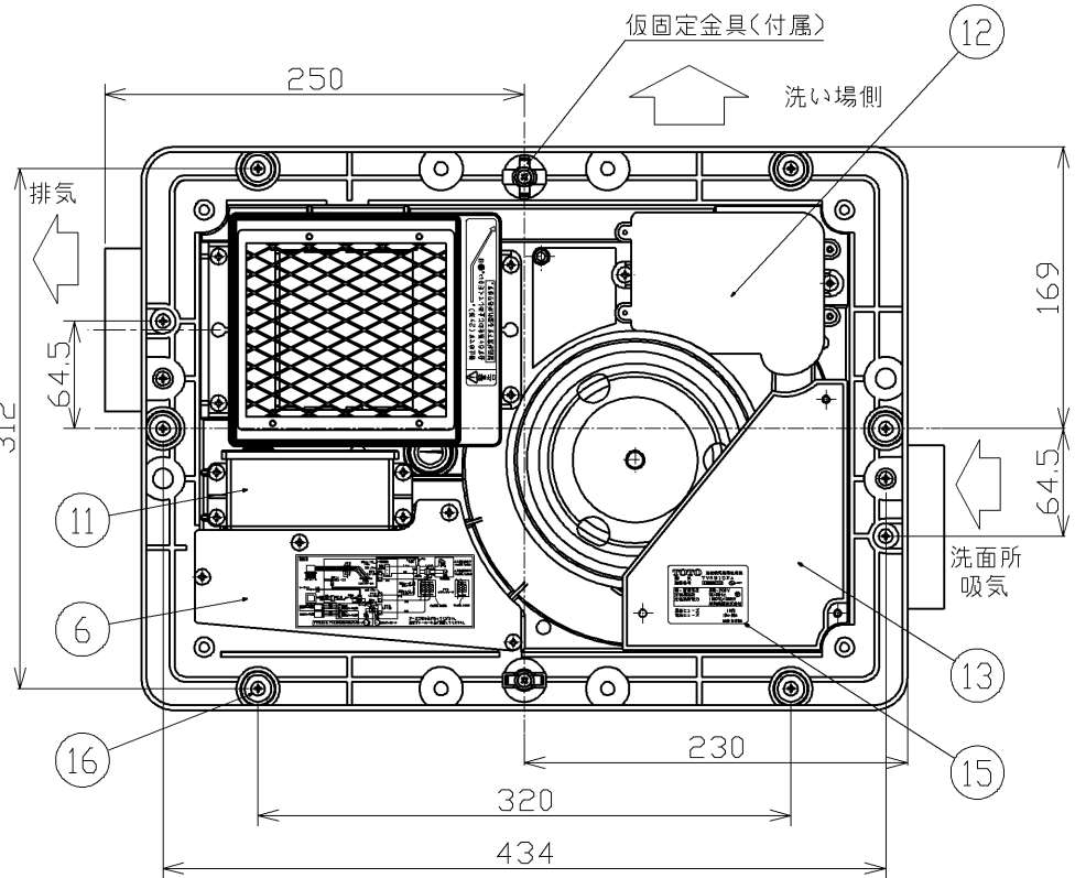
天井取付図 (1:5)
