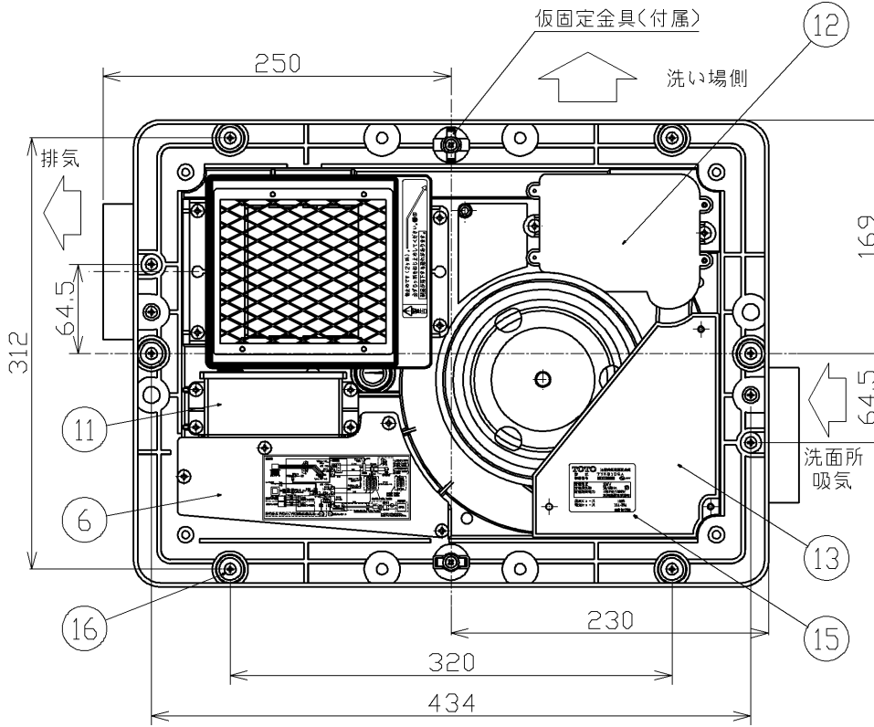
天井取付図 (1:5)
