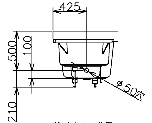
追焚穴あけ位置 ※ステップ下中央
