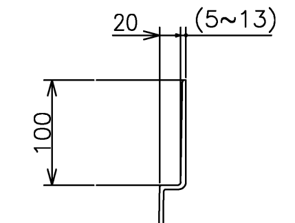
壁のせ部 (防水リム部) 詳細
