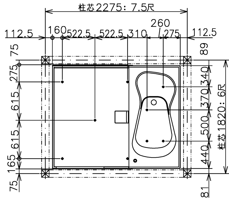
床支持脚位置
