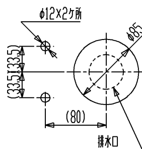
カウンター切込寸法
