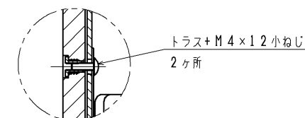
A 部 詳 細 ( S = 1 : 2 )
