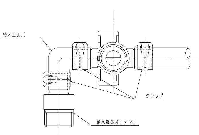
F部詳細図 (S=1:1)
