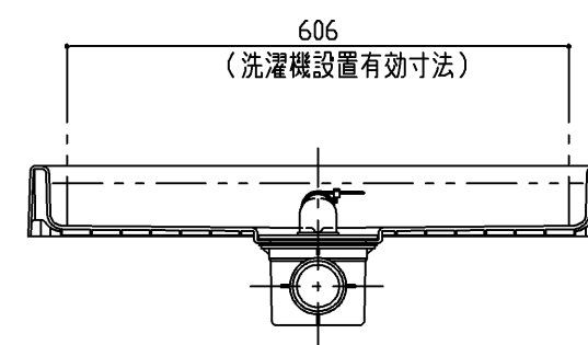
断面B-B
