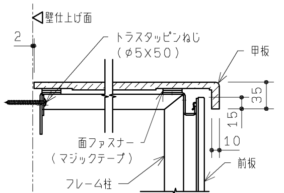
甲板部納まり詳細図（S＝1：5）
