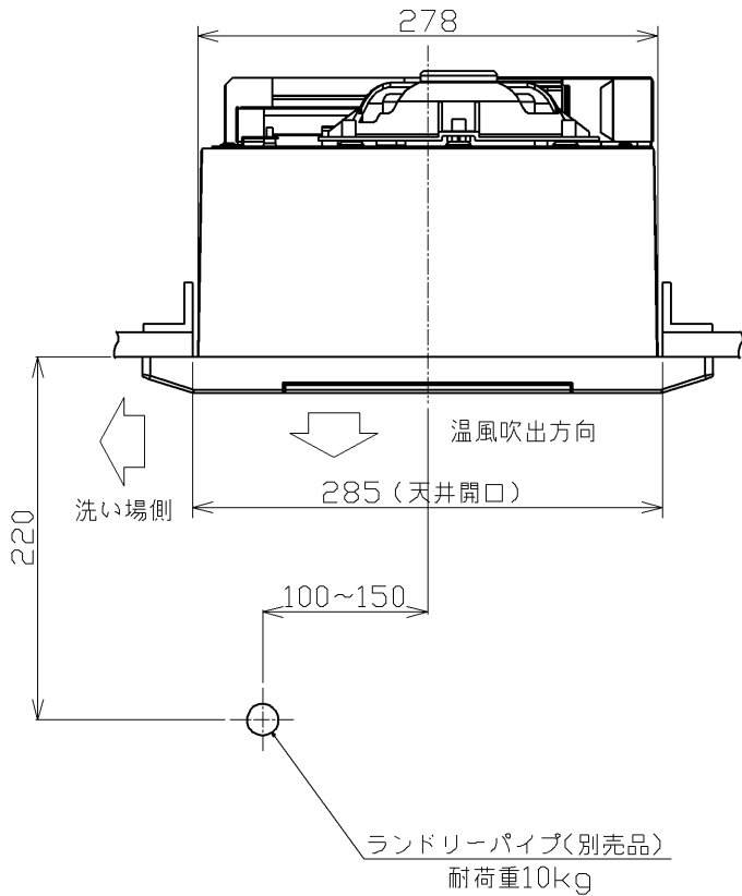
天井取付図 (1:5)
