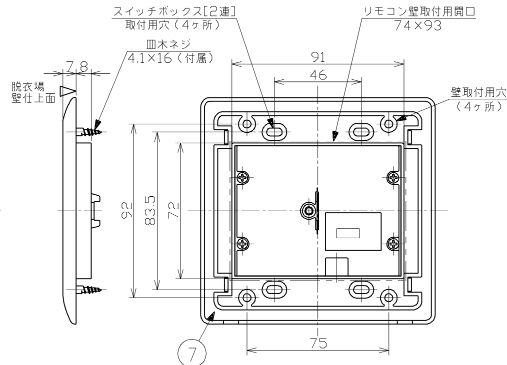
リモコン外観（1：2）
