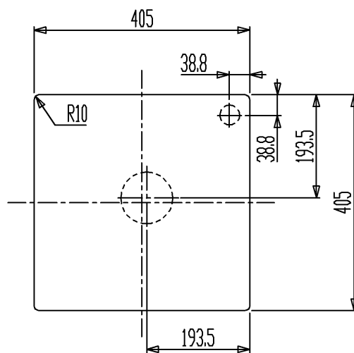
カウンター切込寸法
