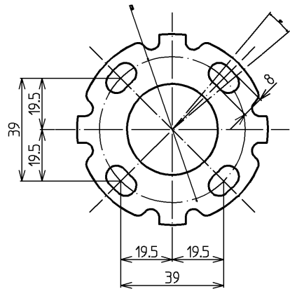
取付座詳細(1:2)
