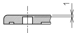
断面 B-B, C-C (1:1)
