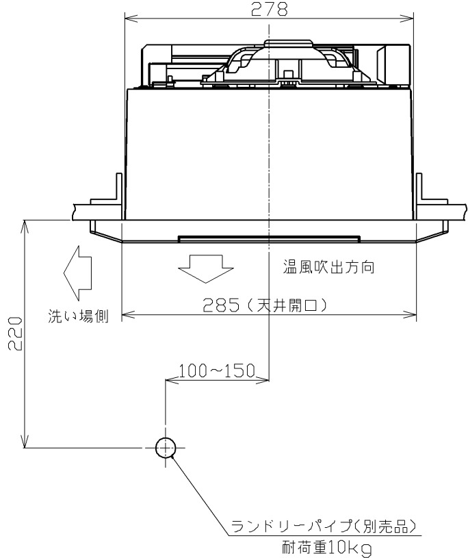
A-A断面
