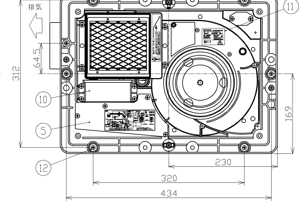
天井取付図 (1:5)
