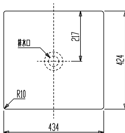
カウンター切込寸法
