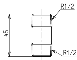
床給水用ニップル
