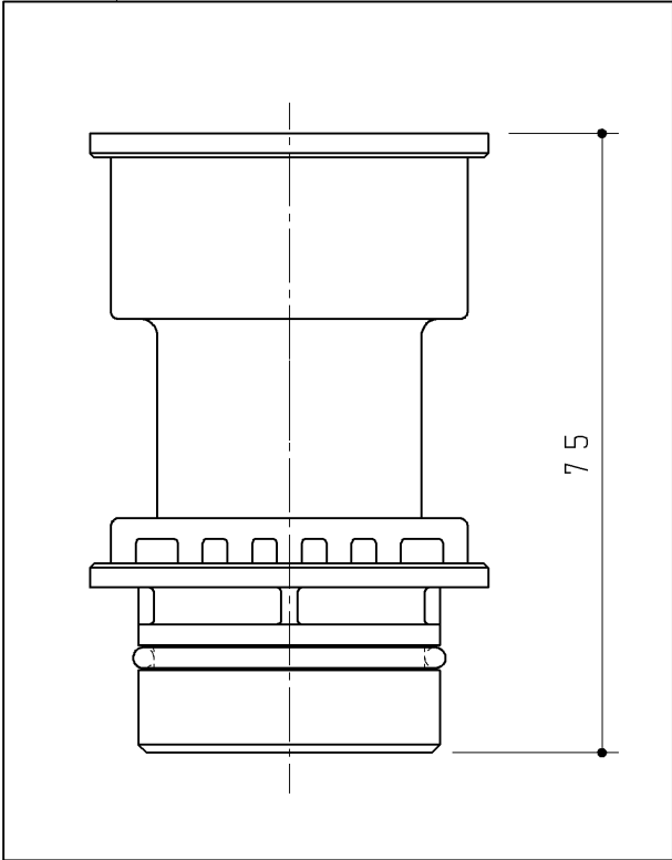
手洗排水横引管（1500）
