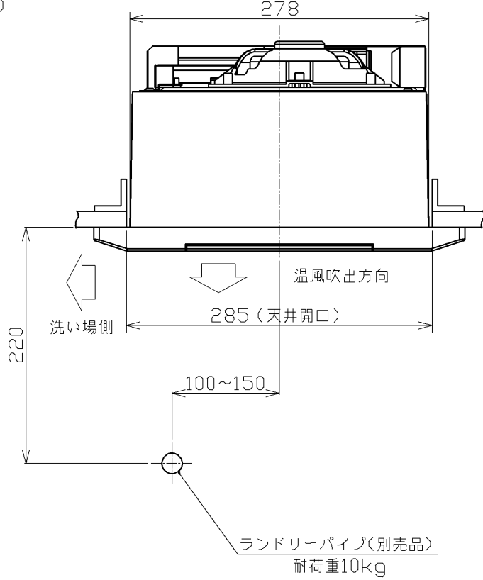
A-A断面
