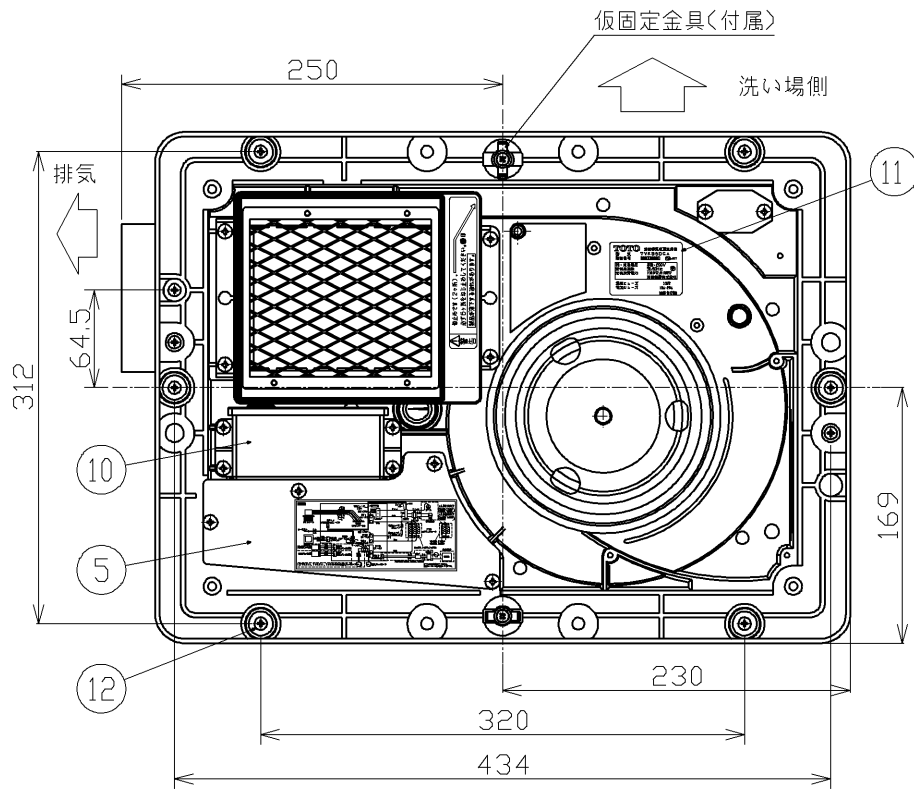
天井取付図 (1:5)
