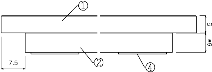
B-B断面図
