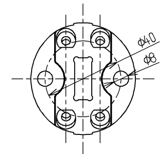
取付座詳細(1:2)
