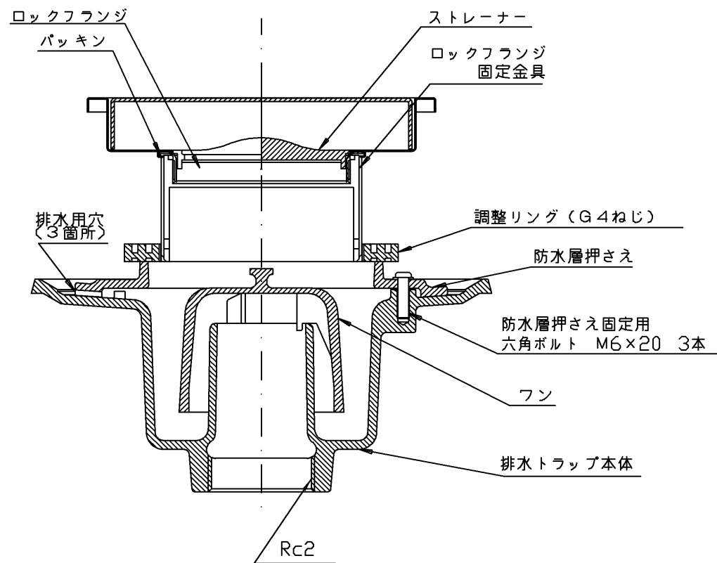
B-B断面 (尺度 フリー)
