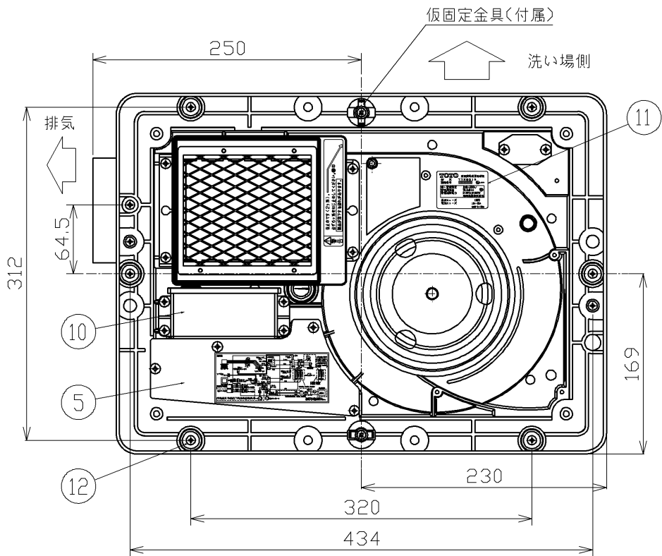
天井取付図 (1:5)
