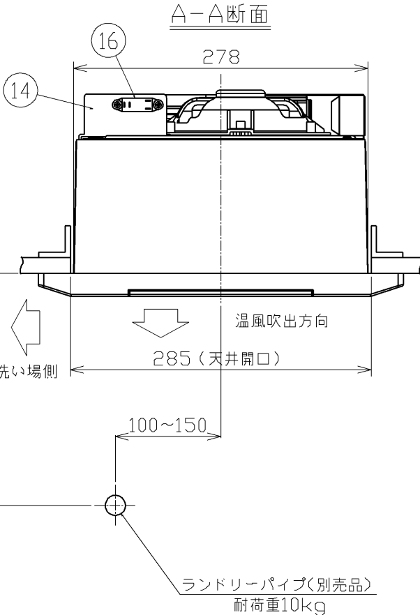
天井取付図 (1:5)
