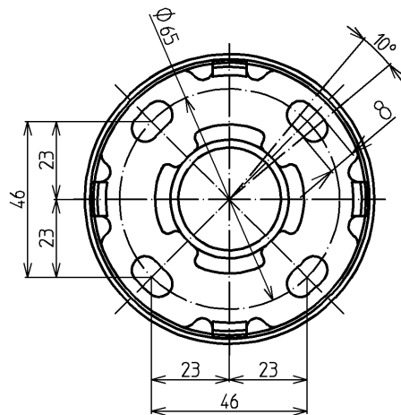
取付座詳細(1:2)
