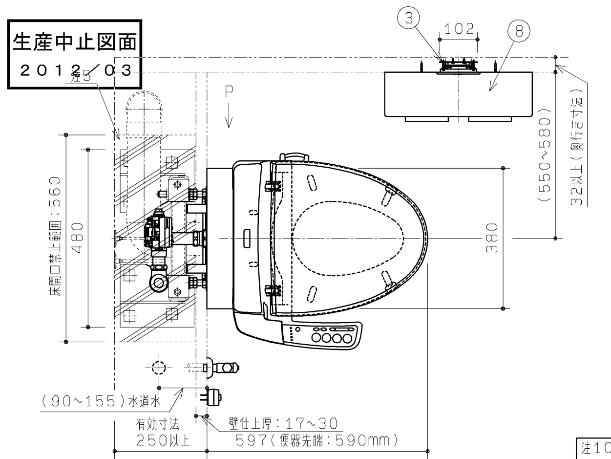
壁掛大便器取付スタンド設置条件
