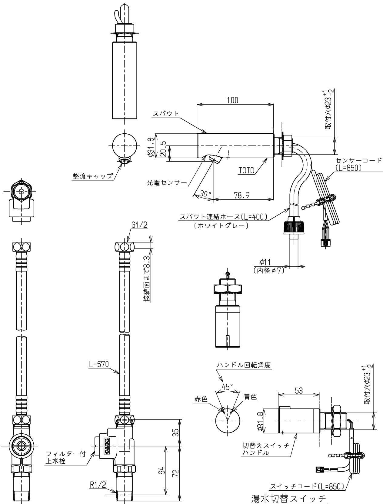
止水栓及びフレキホース
