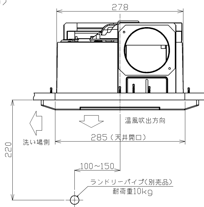
天井取付図 (1:5)
