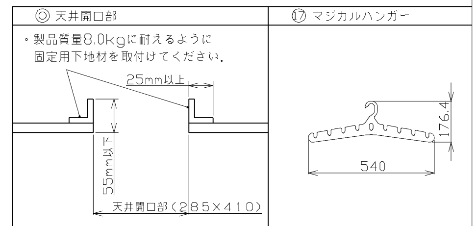
◎ 天井下穴寸法
