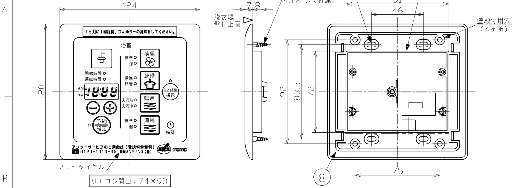
リモコン外観 (1 : 2)
