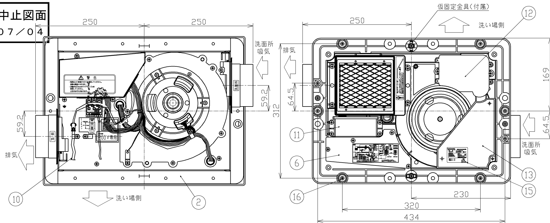
天井取付図 (1:5)
