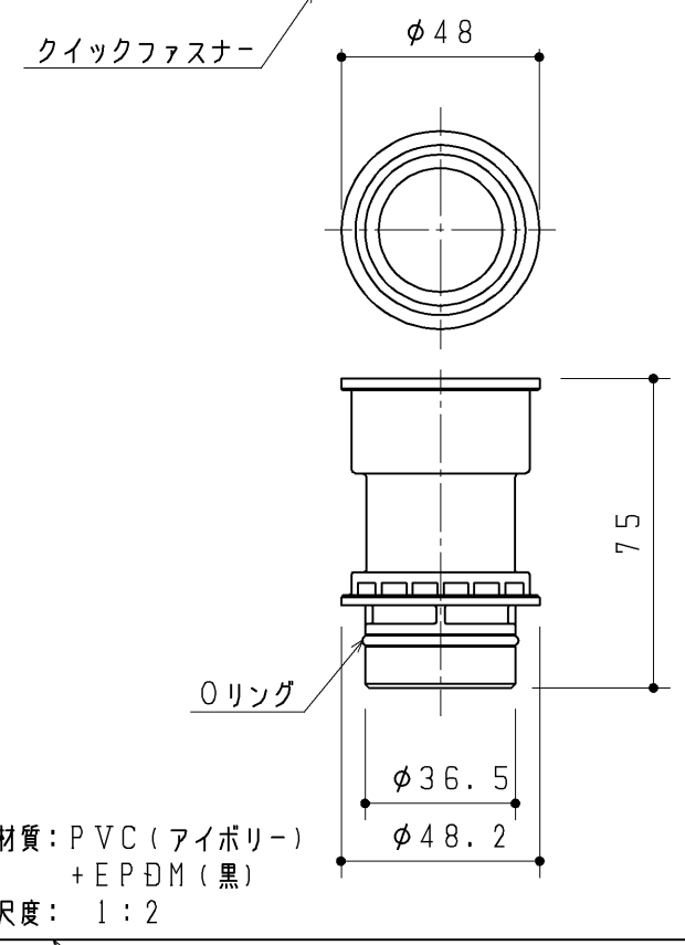
接続継手
