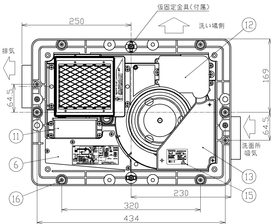
天井取付図 (1:5)
