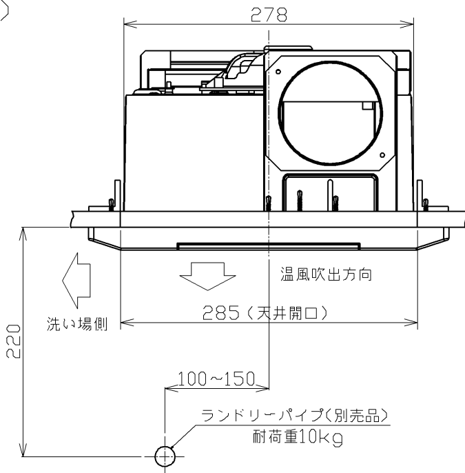
A-A断面
