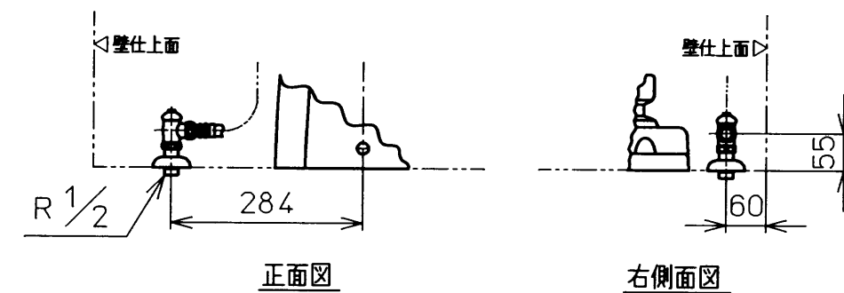
床給水仕様の場合
