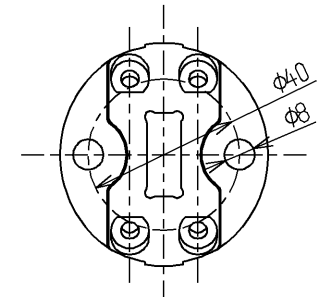
取付座詳細(1:2)
