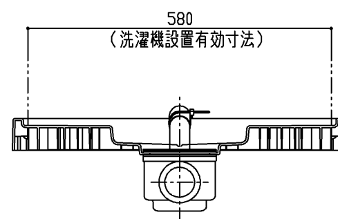
断面B-B
