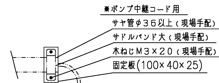
サヤ管固定部詳細図
