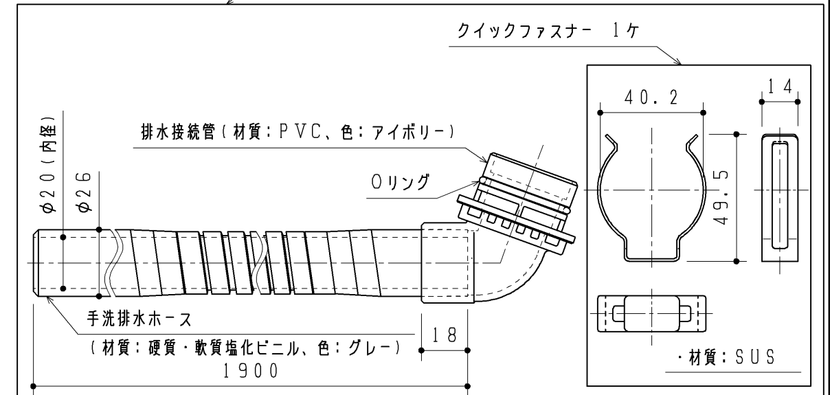
手洗排水ホースセット (床排水)
