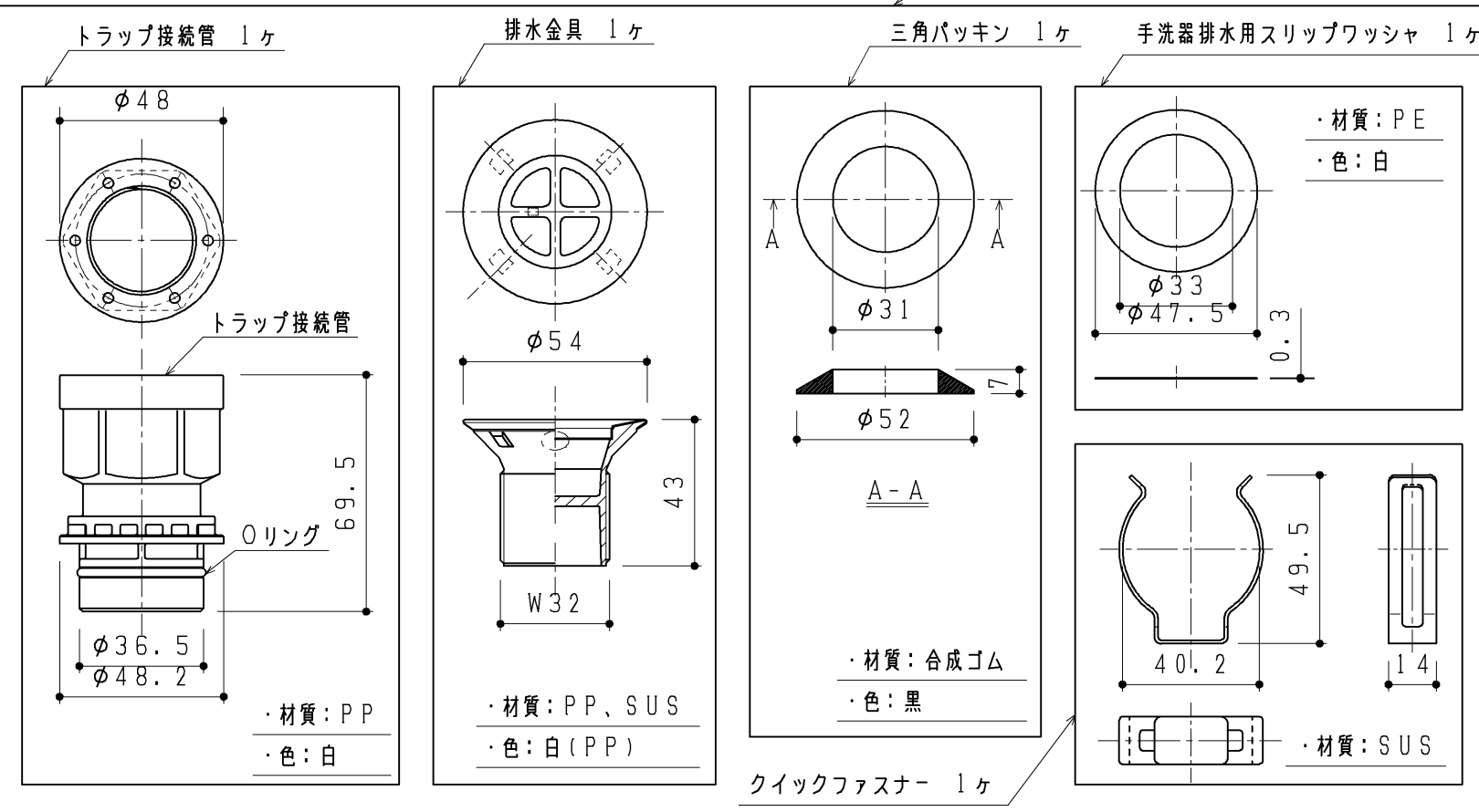
排水金具セット
