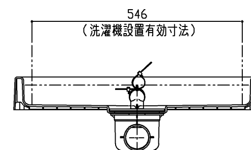
断面B-B
