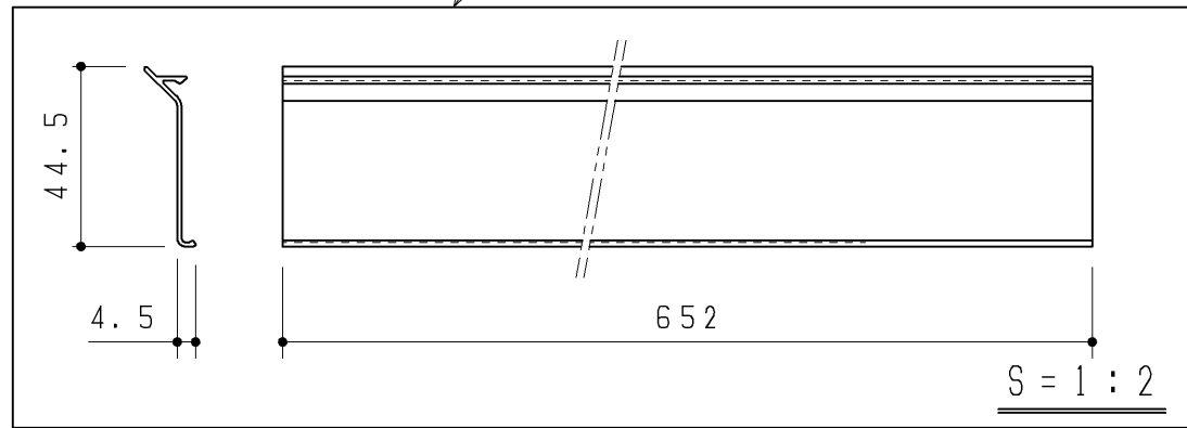
ブラケットカバー
