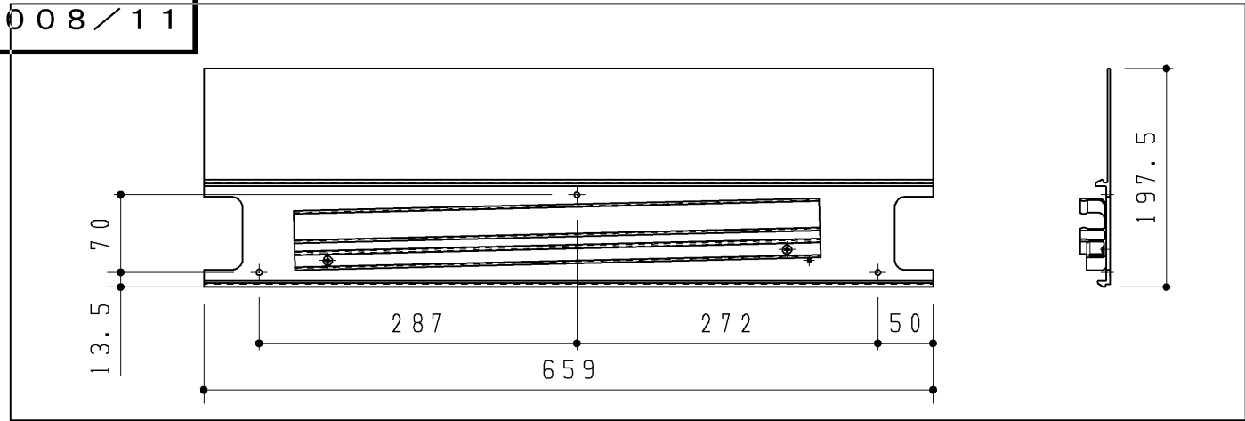
配管カバー
