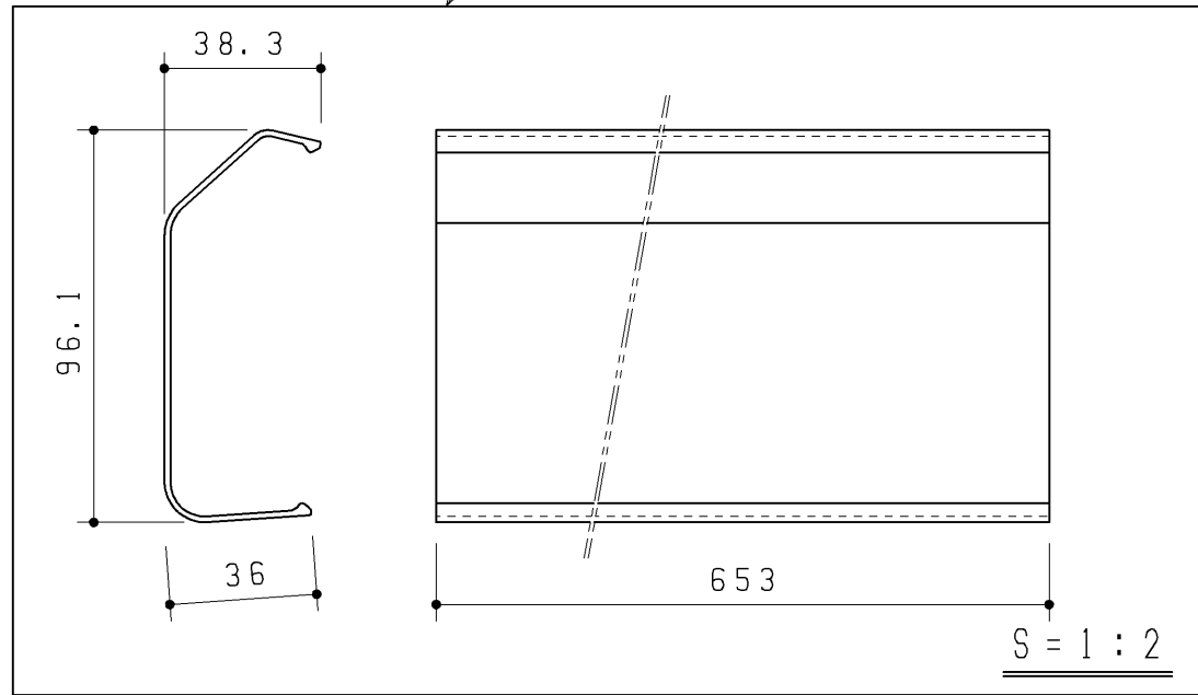
ブラケットカバー
