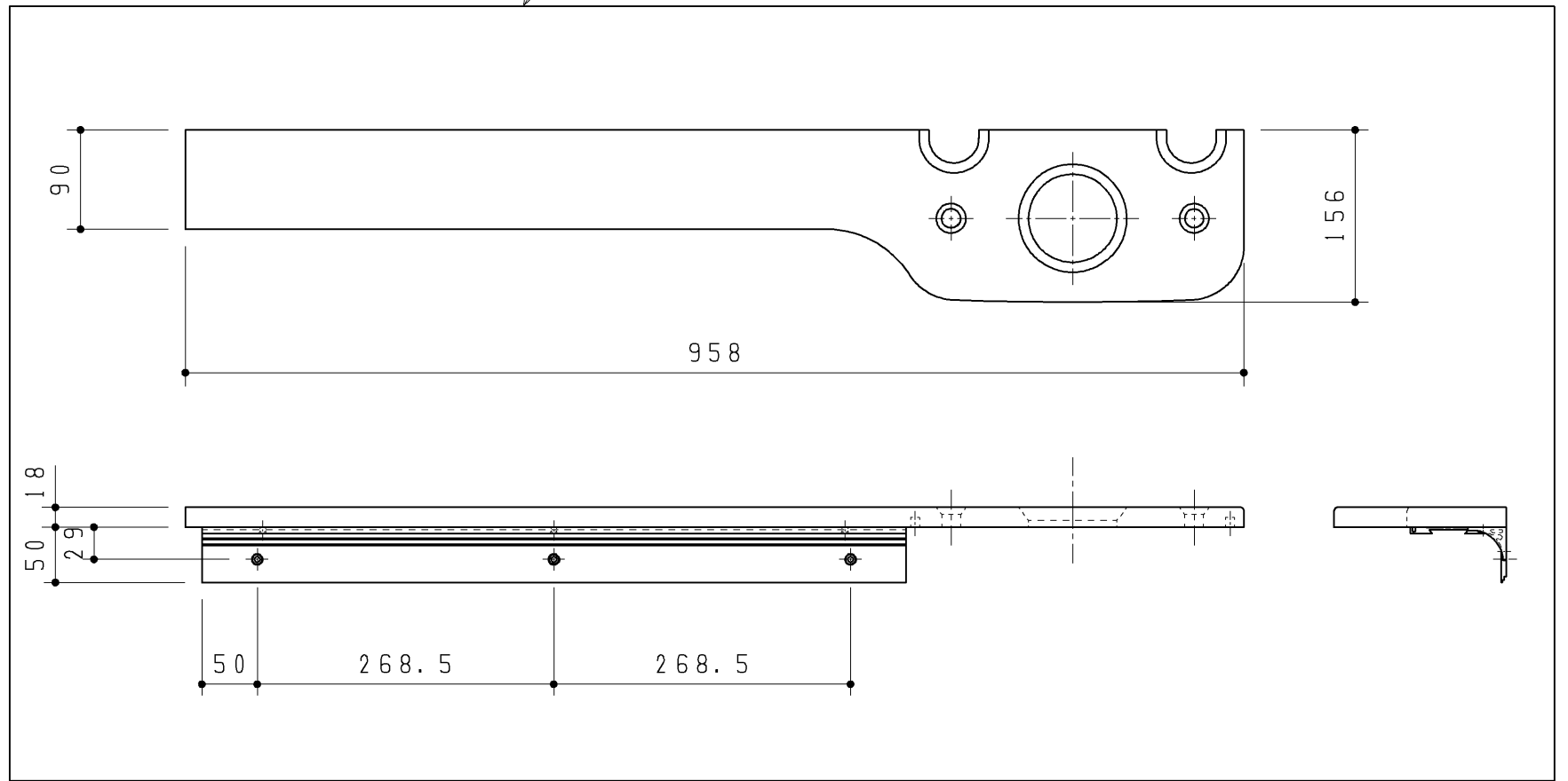
カウンター-R (1200 左右抜き)
