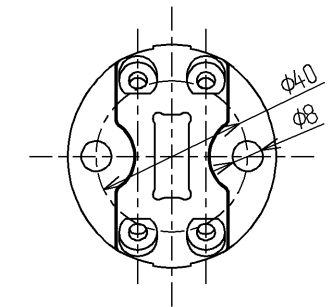
取付座詳細(1:2)
