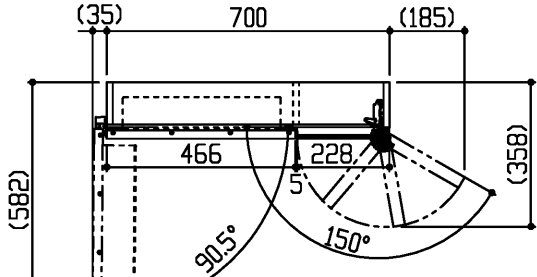
L0125R 軌跡図
