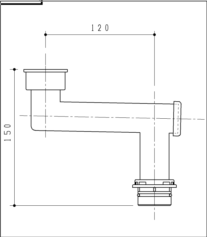
手洗排水横引管（1200）
