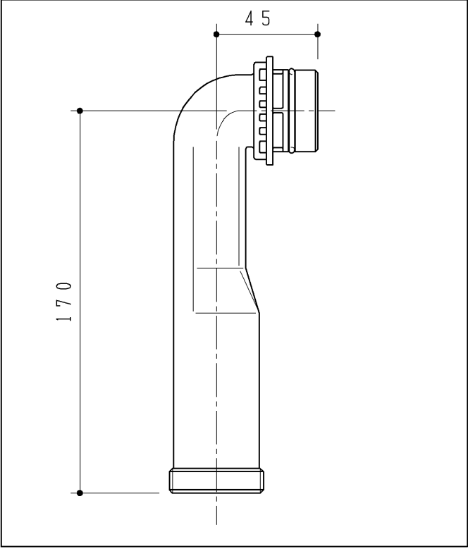
手洗排水縦管（ロング）
