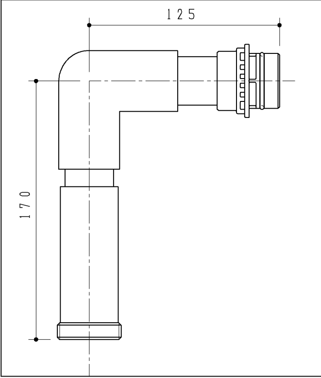
手洗排水横引管（1200）
