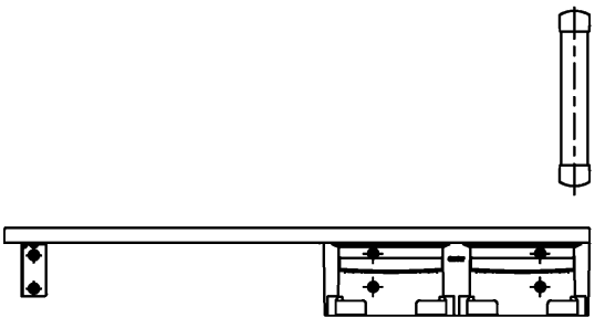
右壁設置の場合(1:10)
