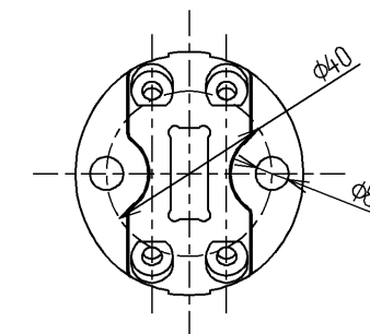
取付座詳細(1:2)
