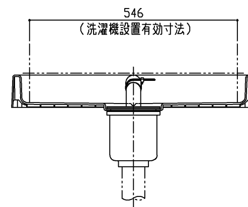
断面B-B
