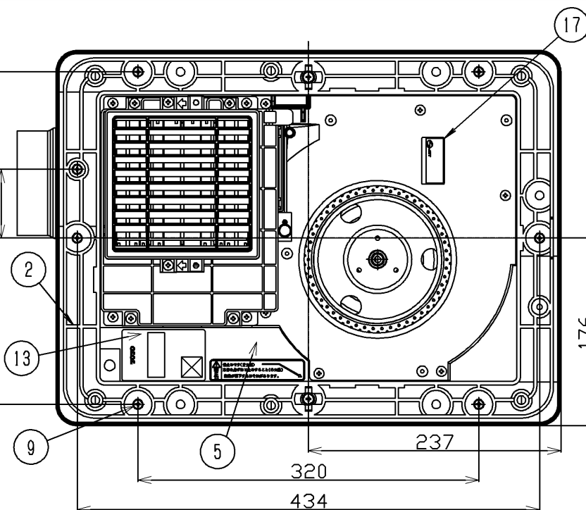
A-A断面
