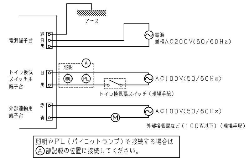
結線図
