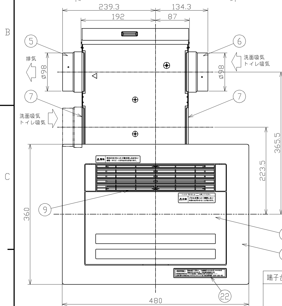
天井取付図 (1:5)
