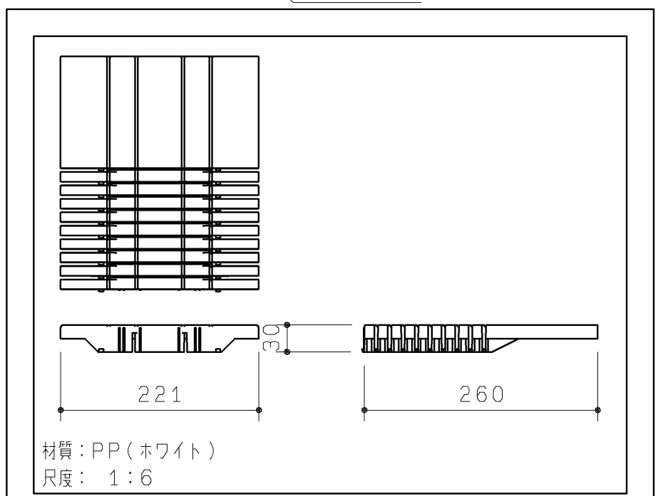
棚板（2ヶ）
