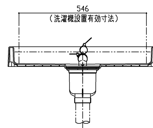
断面B-B
