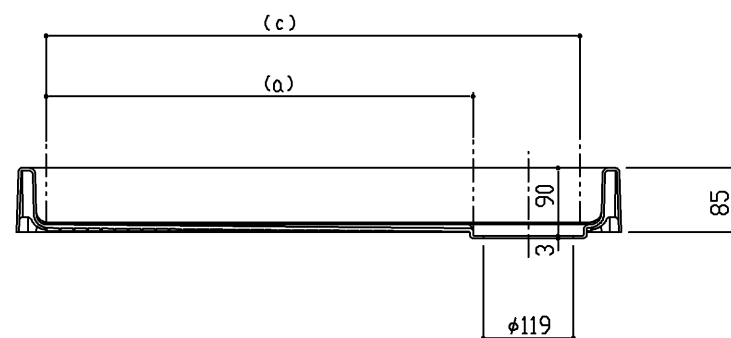
断面A-A
