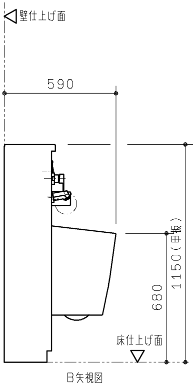
B矢視図
