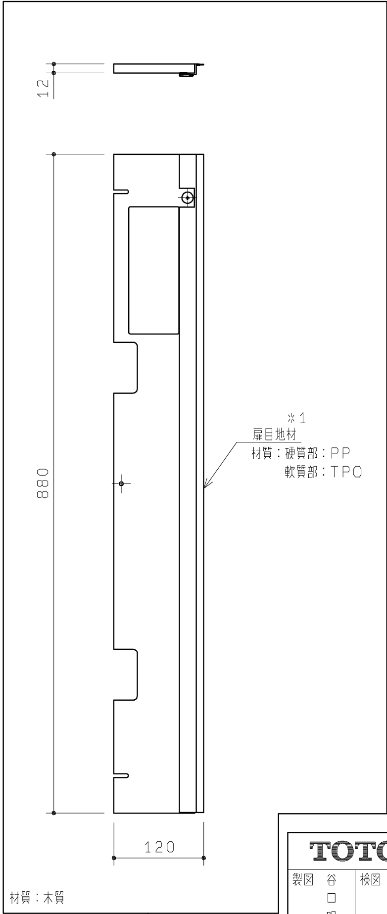
裏扉セット
